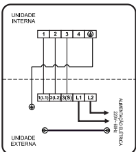
Esquema de ligação de unidades 12/18/24.000 Frio / 12/18/24.000 Quente/Frio - 220V
