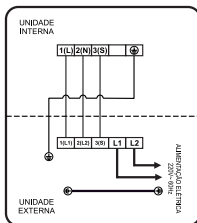
Esquema de ligação de unidades 9.000 Frio / 9.000 Quente/Frio - 220V
